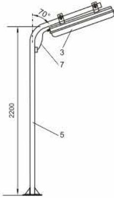
法兰式(F)
