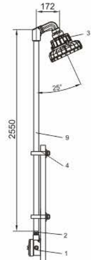
护栏式(h2)
