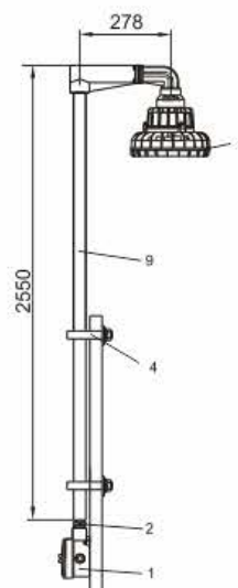
护栏式(h1)
