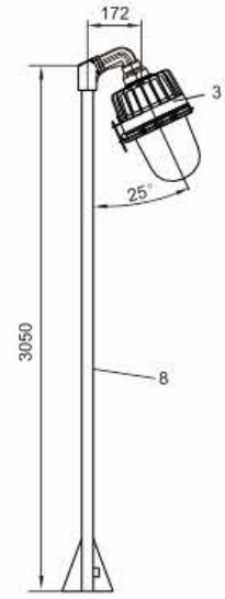
法兰式(F2)
