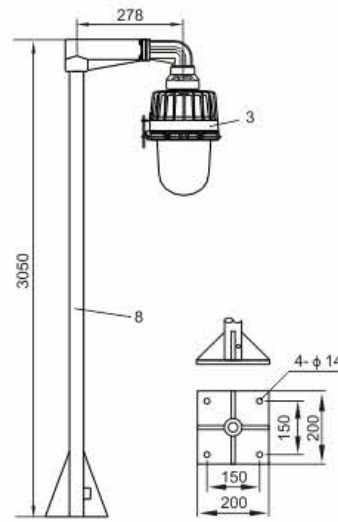
法兰式(F1)
